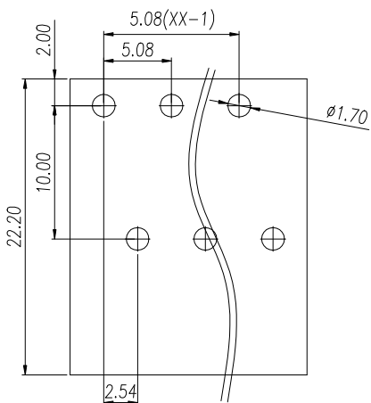
P.C.B. LAYOUT
